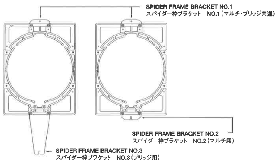
BRACKET NO. ブラケット 部品番号一覧
