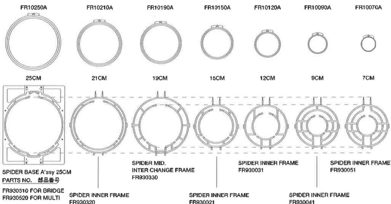
PARTS NO. 部品番号
